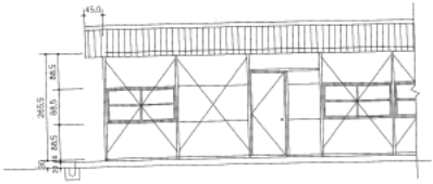
⊕ 正向立面圖
