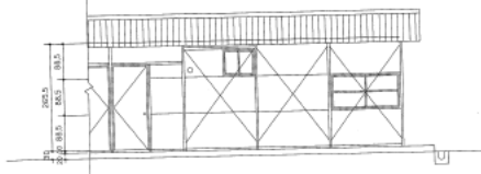
⊕ 背向立面圖
