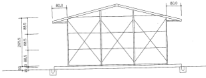
⊕ 側向立面圖
